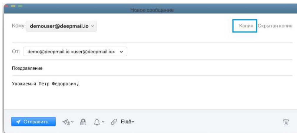
Рисунок 98 – «Копия»
