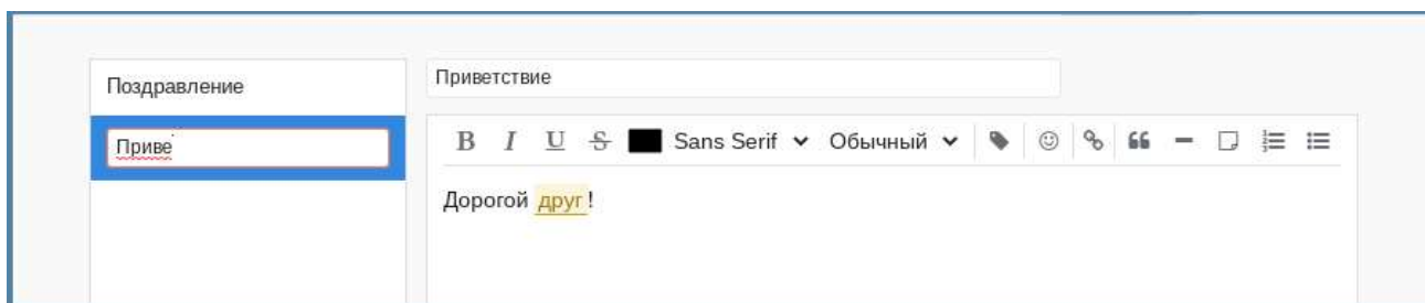
Рисунок 114 – Редактирование наименования
