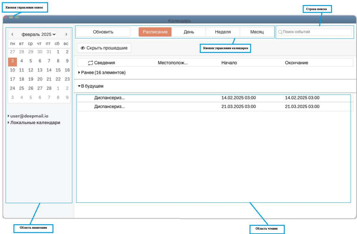
Рисунок 222 – Окно календаря
