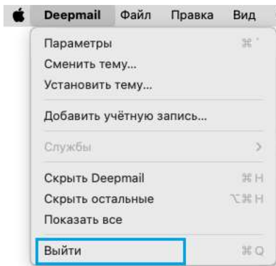
Рисунок 260 – Операция «Выйти»
