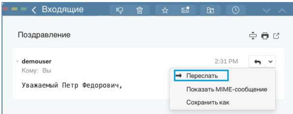
Рисунок 147 – Операция «Переслать»
