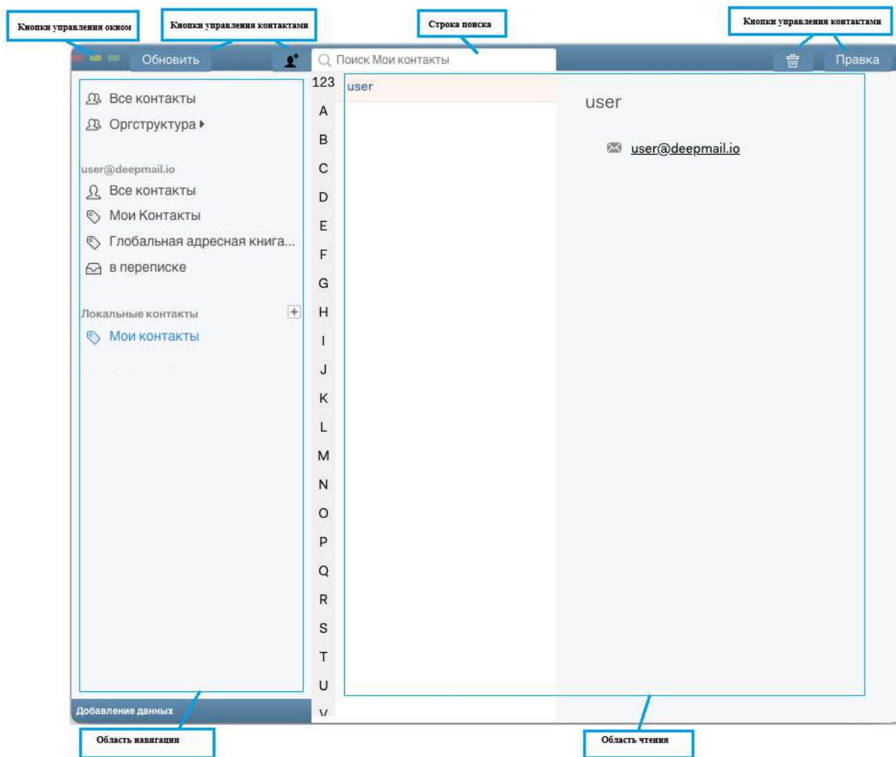
Рисунок 197 – Окно «Контакты»
