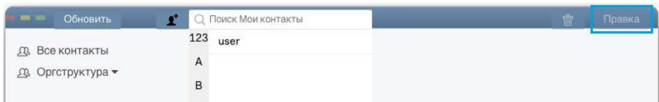
Рисунок 215 – Кнопка «Правка»
