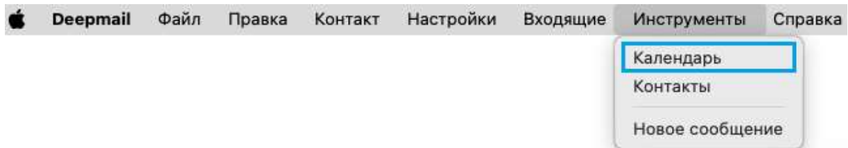
Рисунок 221 – «Календарь»
