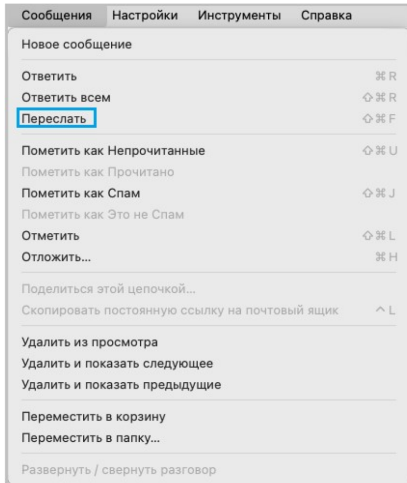
Рисунок 144 – Операция «Переслать»
