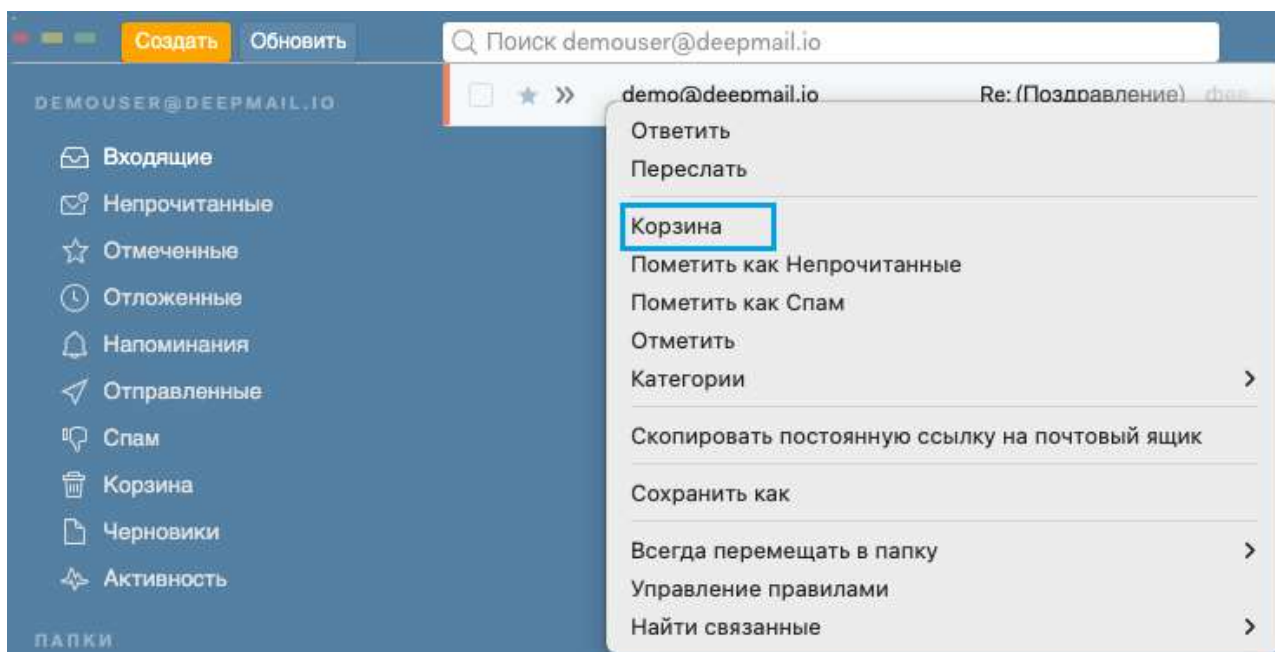
Рисунок 180 – Операция «Корзина»
