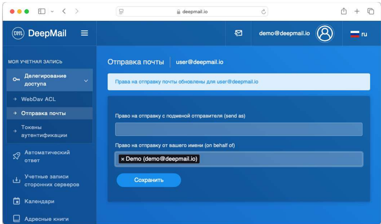
Рисунок 137 – Указание адреса
