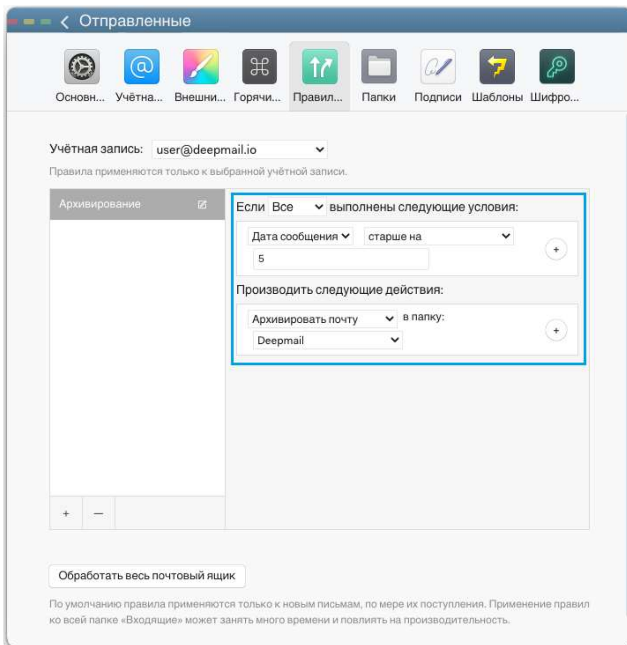
Рисунок 194 – Условия архивирования
